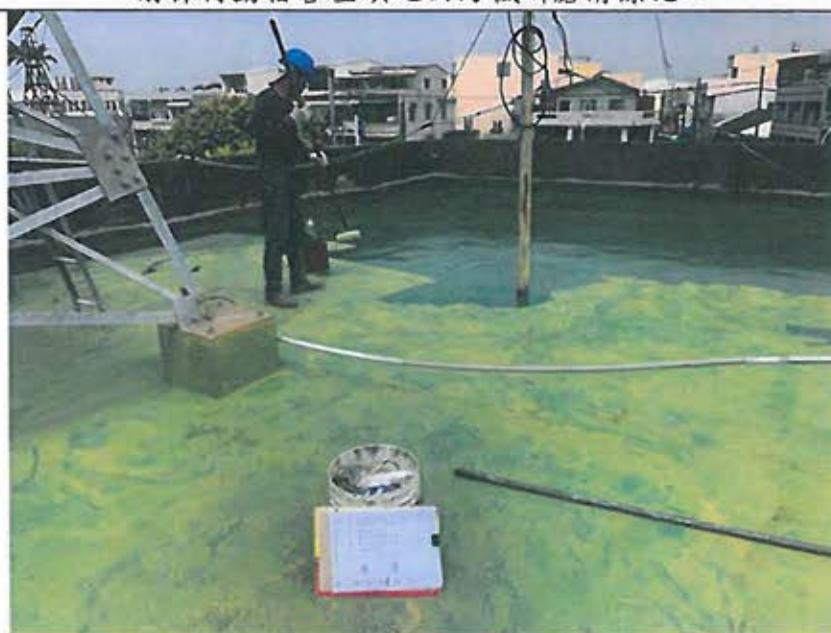
前棟待勤宿舍屋頂地面防水 PU 底漆施工
