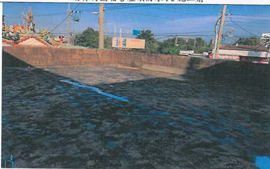
前棟待勤宿舍屋頂防水 PU 底漆施工
