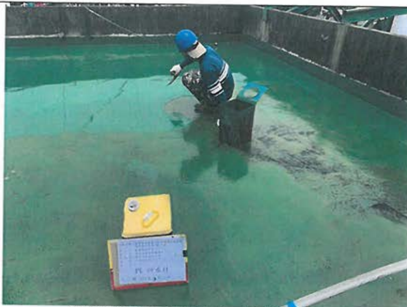
前棟待勤宿舍屋頂地面防水 PU 中才施工
