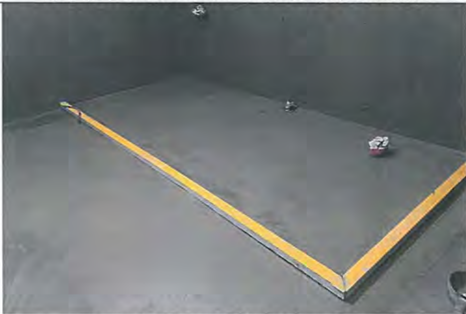
3樓待勤鹽洗室牆壁地面防水塗刷施工
