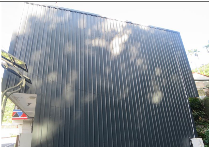
待勤宿舍外牆釘封烤漆板施工後
