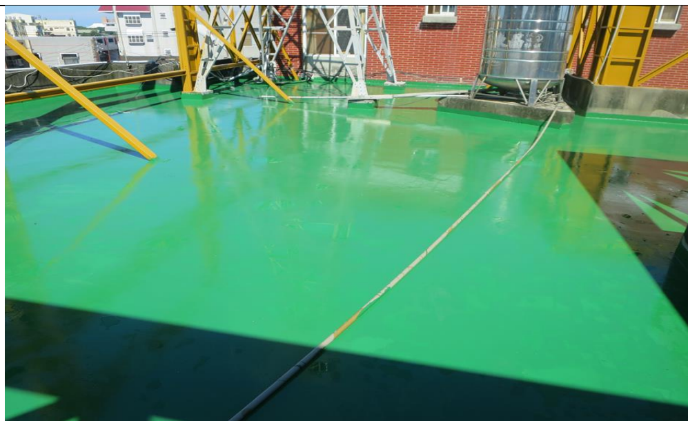
屋頂地面施作防水 PU 施工後
